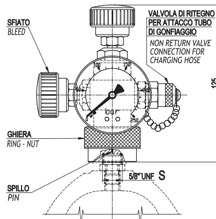
Riduzioni per attacchi speciali valvole gas Adapter for special valve connection
