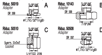
Riduzioni per attacchi speciali valvole gas Adapter for special valve connection
